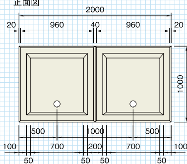
正面図
