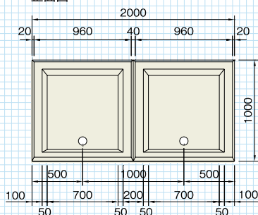
正面図
