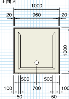
正面図
