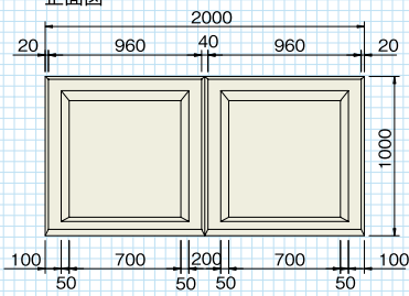
正面図
