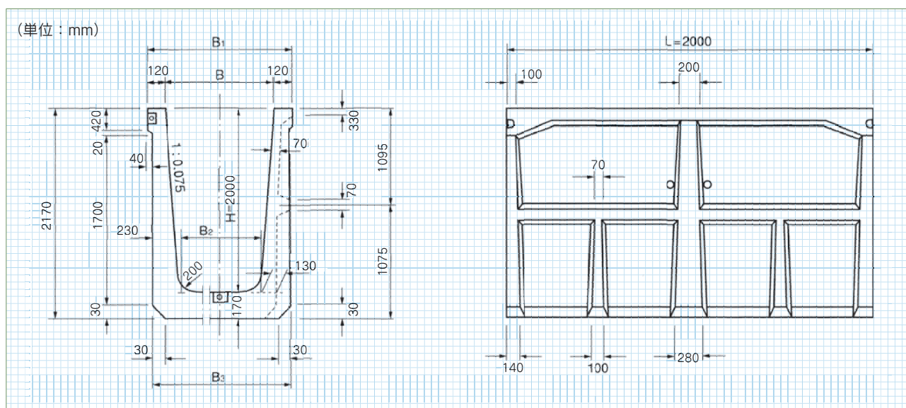
製品寸法図
