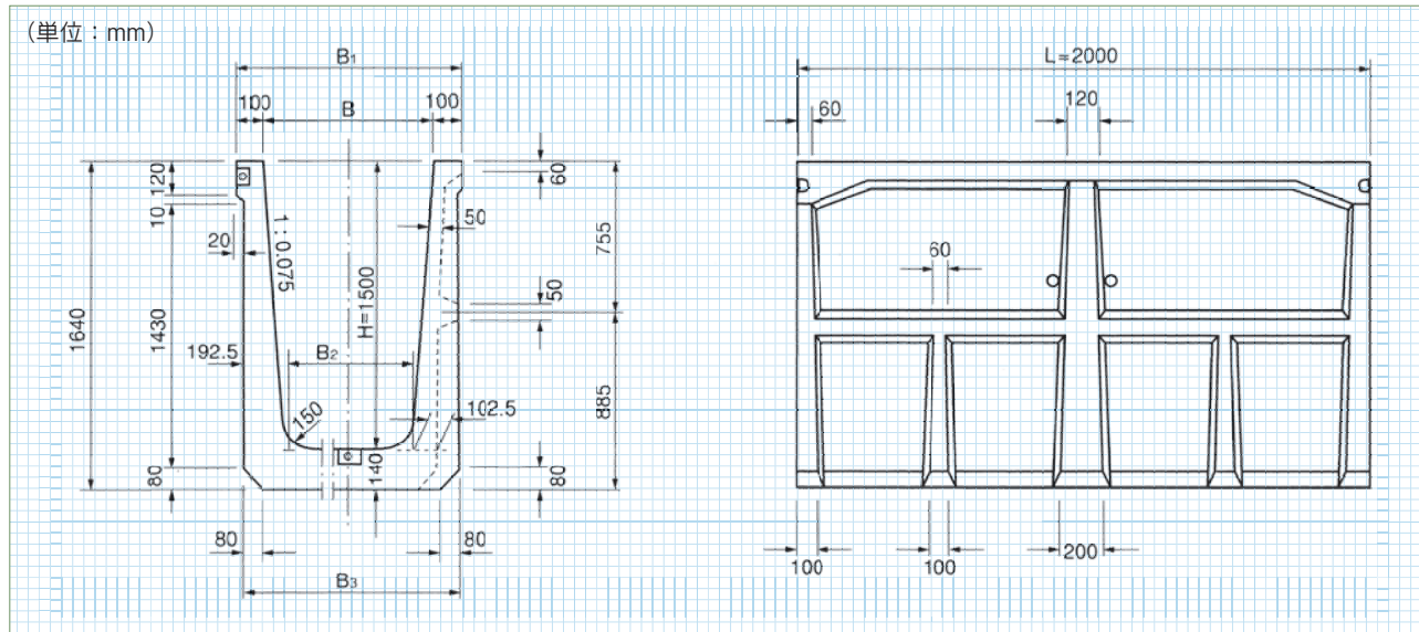
製品寸法表
