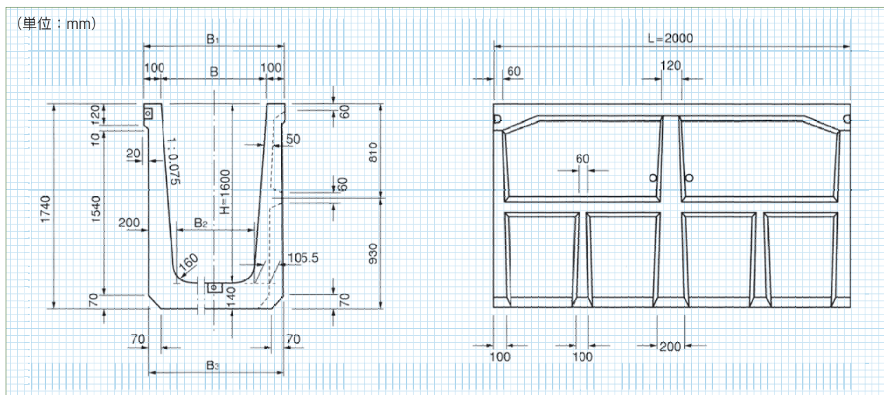
製品寸法表
