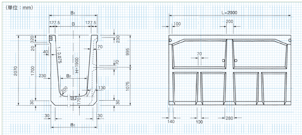
製品寸法表
