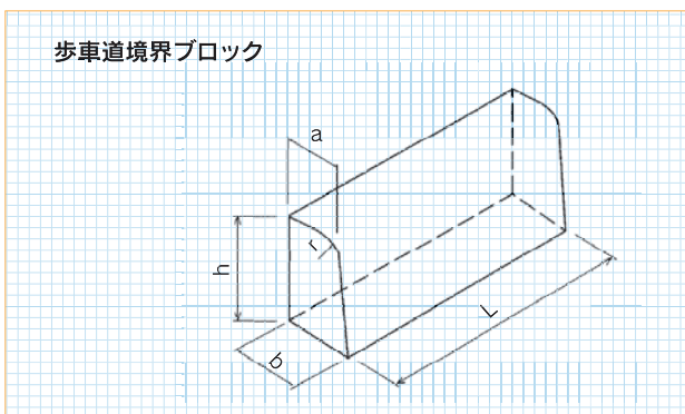
製品寸法図
