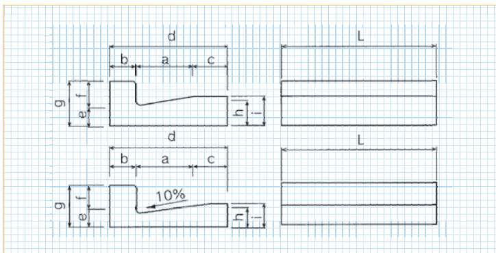
製品寸法図
