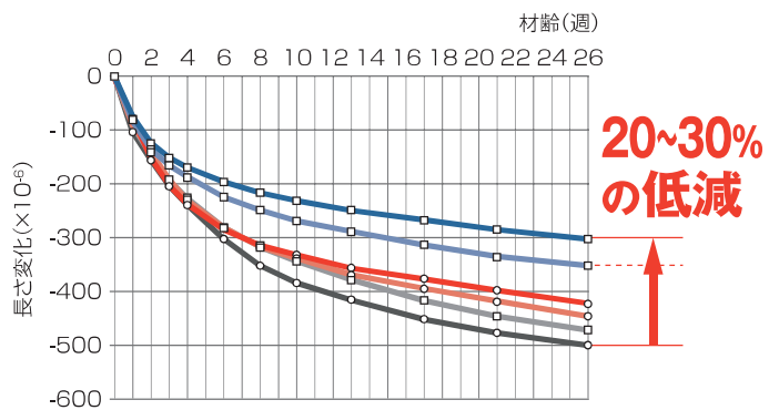
長さ変化試験結果(W/B=50% 骨材として海砂・硬質砂岩を使用) 試験方法(JIS A 1129-3)「モルタル及びコンクリートの長さ変化試験方法」
