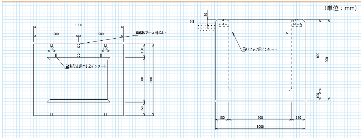
■航空局規格(A-b型) (参考重量=1,078kg)
