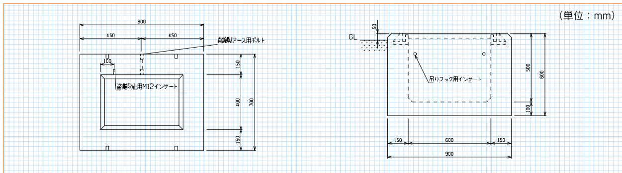
■航空局規格(B型) (参考重量=606kg)
