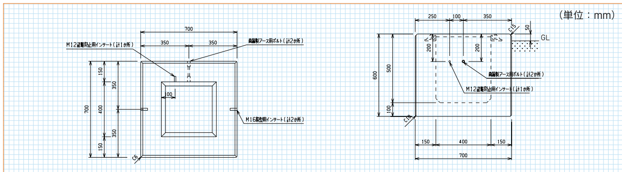
■航空局規格(C-a型) (参考重量=320kg)
