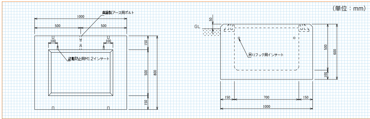
■航空局規格(A-a型) (参考重量=1,056kg)
