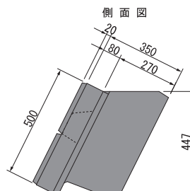
側面図
