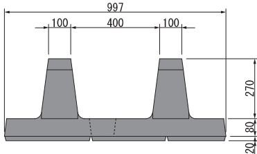
正面図
